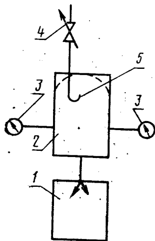
1—испытуемый насос; 2—измерительная камера; 3—измерительные преобразователи давления; 4—насос; 5—напускная трубка
