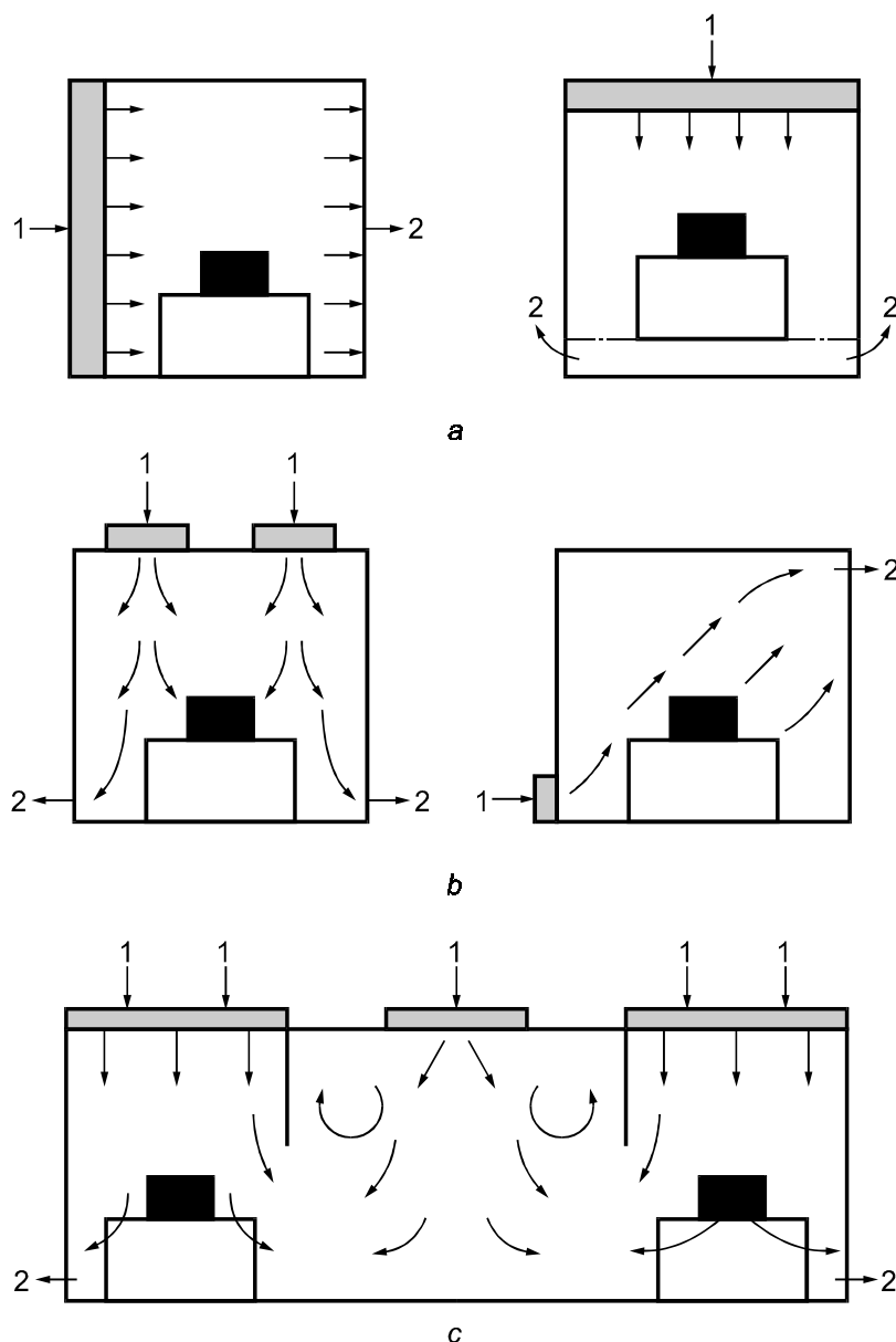
а — однонаправленный поток воздуха; б — неоднаправленный поток воздуха; с — смешанный поток воздуха; 1 — приточный воздух; 2 — вытяжной воздух
