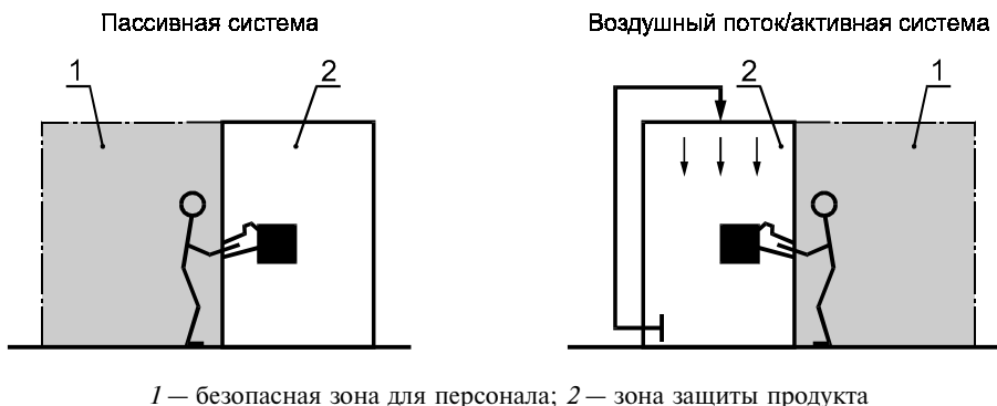
Рисунок А.5 — Принципы организации чистых зон с использованием физического барьера защиты продукта и персонала
