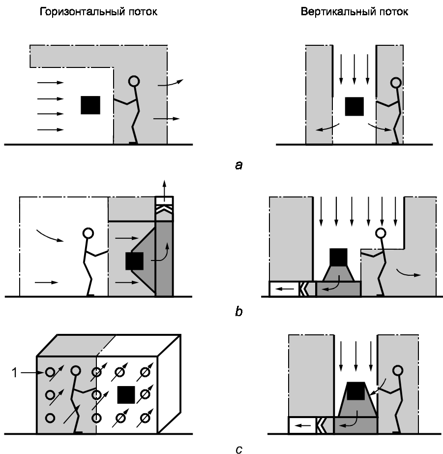
a — защита продукта; b — защита персонала и окружающей среды; c — защита персонала, продукта и окружающей среды; l — направление потока перпендикулярно к плоскости рисунка
